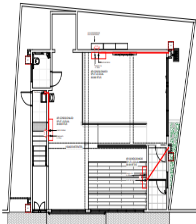
1 PLANTA BAIXA PAVIMENTO TÉRREO - AR CONDICIONADO ESCALA 1:50
